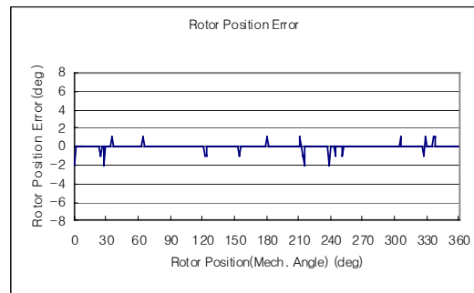
Fig. 8 Rotor position error
